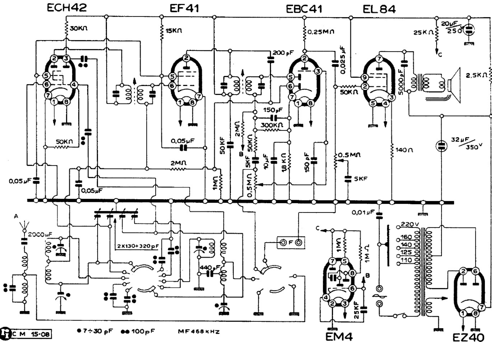
TRANS CONTINENTS RADIO TV - Mod. PD 28 con gruppo VAR
